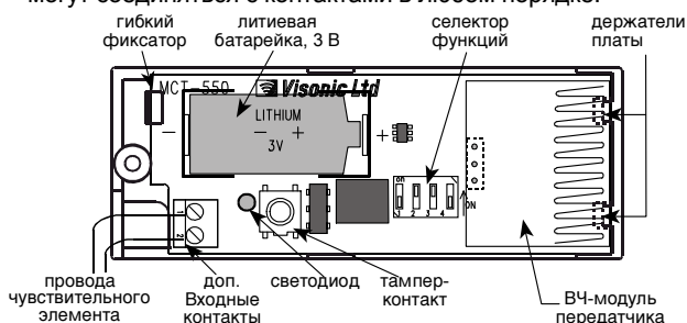
Рис. 11 - Плата
