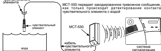
Рис. 5 - Применение датчика МСТ-550
